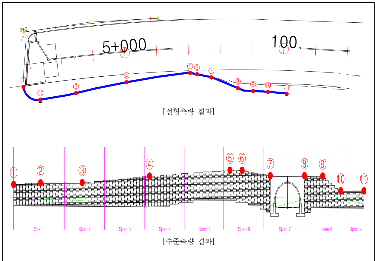
【그림 7.3.5】 선형 및 수준측량 결과
