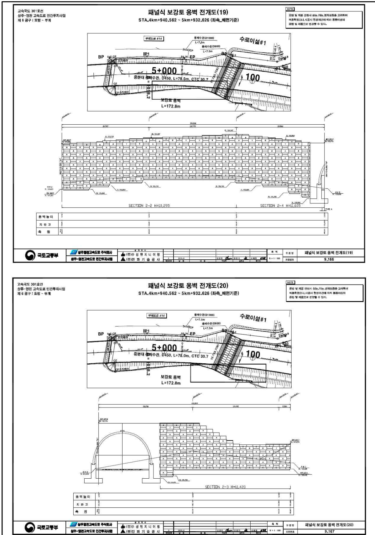
【그림 7.1.4】전개도(계속)
